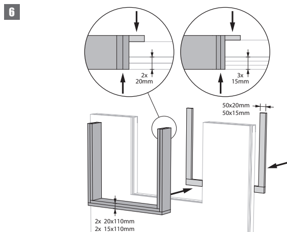
6. Alternatief kan de beplating in de dagkant getrappt uitgevoerd worden.
