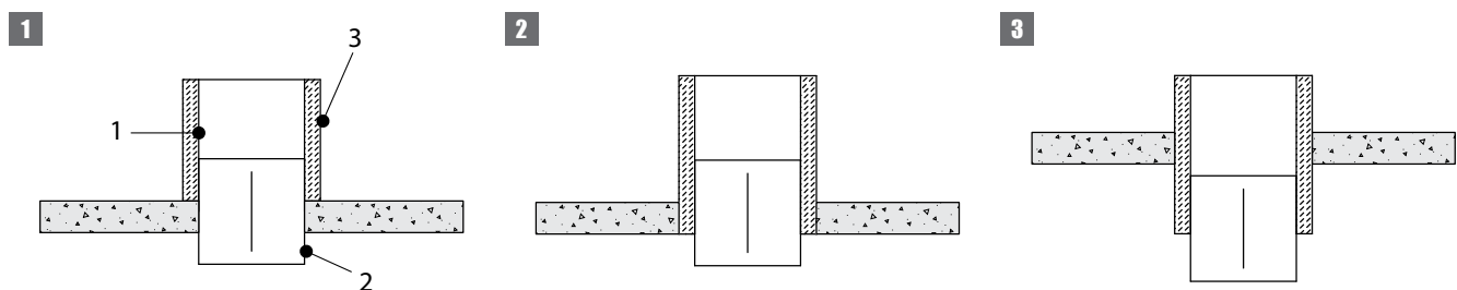
1. Conduit - 2. Volet - 3. Isolation thermique assurée par le conduit
